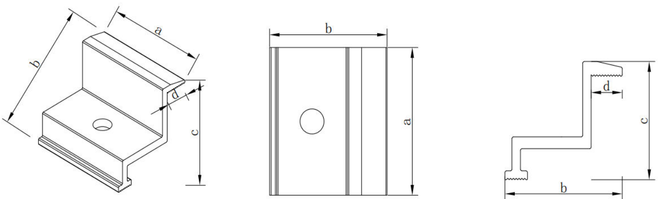
Fig. 5 Clamp
