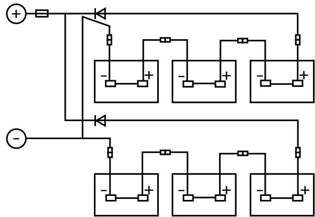
Gecombineerde schakeling
