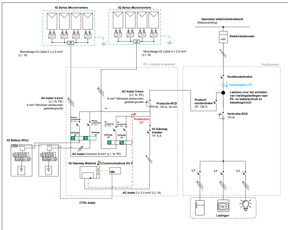
Afbeelding 4: Eénfasig IQ7/IQ8 Series PV (meerdere takken) en IQ Battery 5P (serieschakeling) systeemdigram
