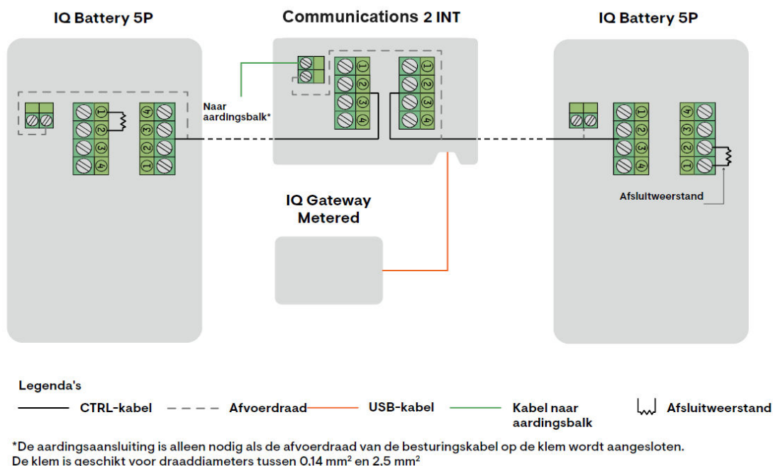
Afbeelding 12: Draadvolgorde CTRL-kabel 2
