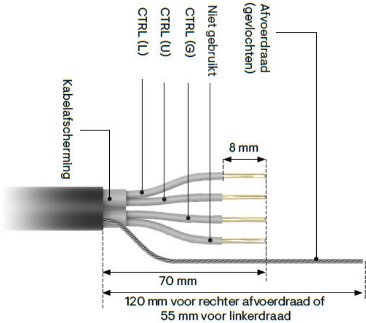
Afbeelding 9: CTRL-kabel draadstripgeleiding
