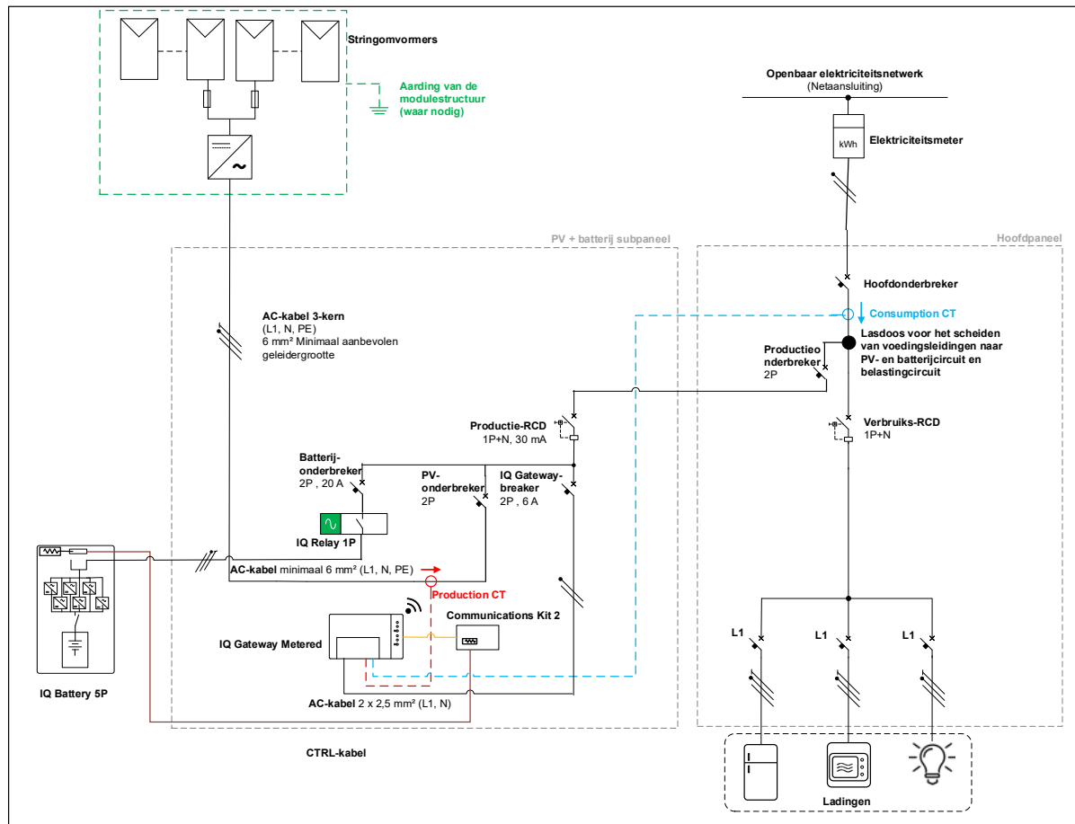
Afbeelding 5: Eenfasige stringomvormer PV en IQ Battery 5P systeemdijagram
