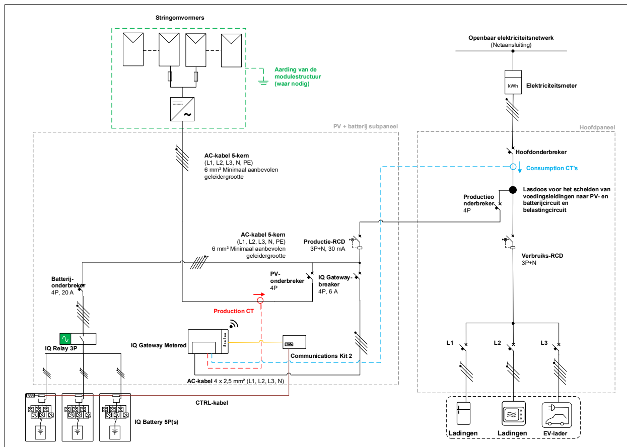
Afbeelding 8: Driefasig stringomvormer PV en IQ Battery 5P systeemdigram
