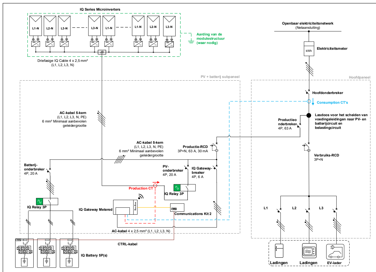
Afbeelding 7: Driefasig IQ7/IQ8 Series PV en IQ Battery 5P systeemdigram
