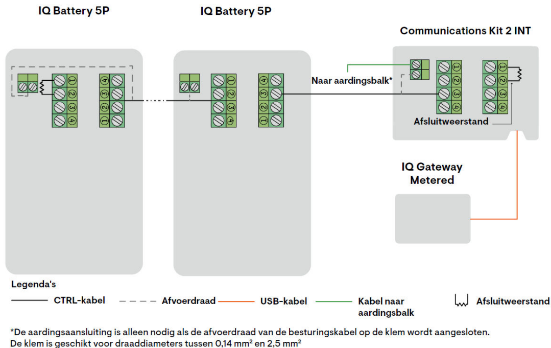
Afbeelding 11: Draadvolgorde CTRL-kabel 1
