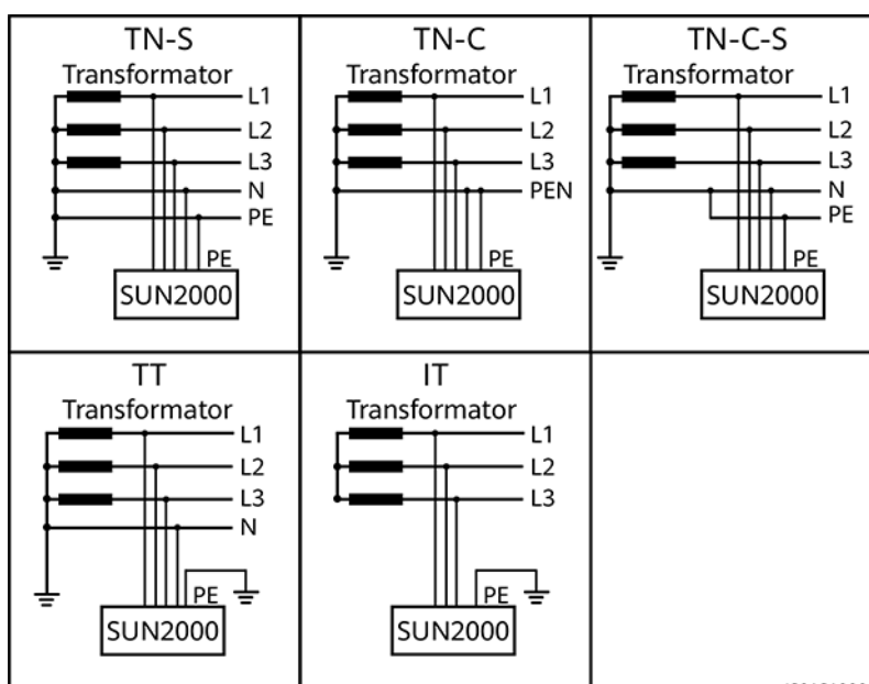
Afbeelding2-6 Ondersteunde elektriciteitsnetten
