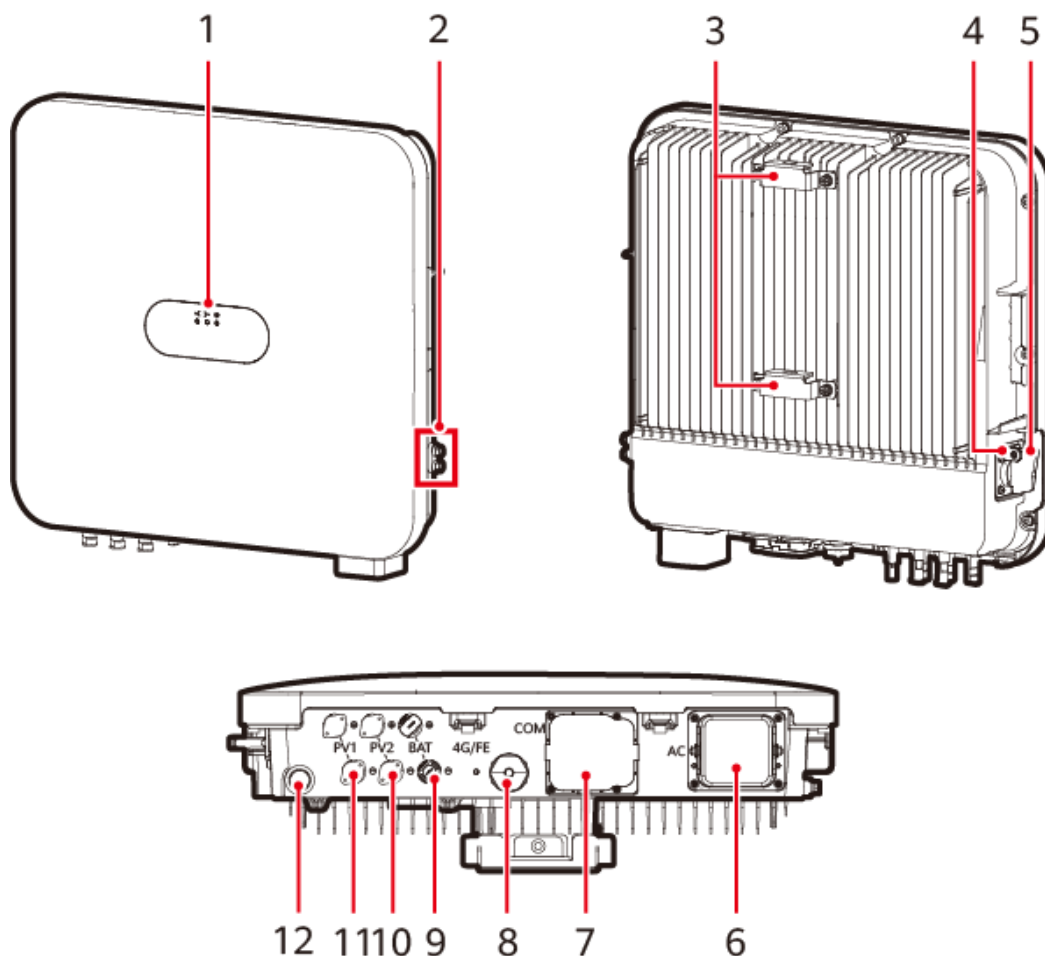
Afbeelding2-7 Uiterlijke kenmerken
