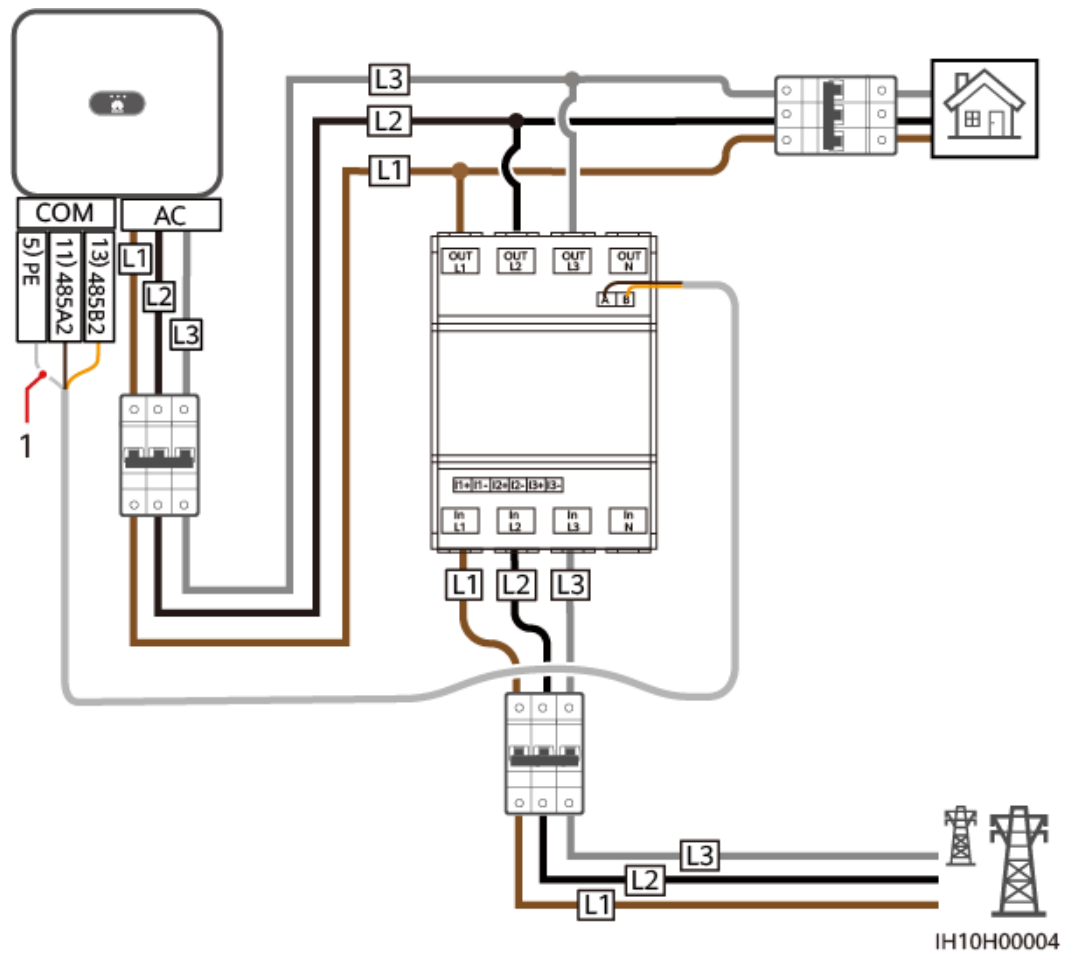
Afbeelding5-24 Driefasige, driedraadse directe aansluiting (Smart Dongle-netwerk)
