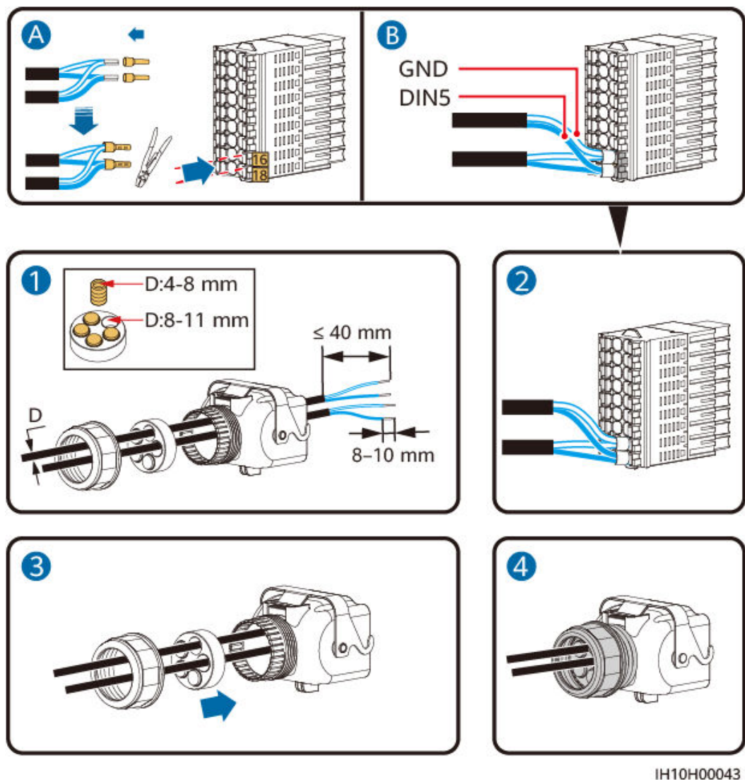
Afbeelding5-39 Kabels installeren
