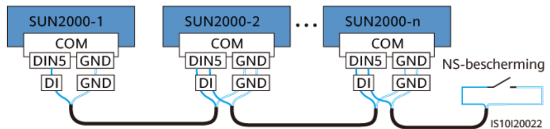
Afbeelding5-38 Gecascadeerde omvormers aansluiten op de NS-beschermingsschakelaar
