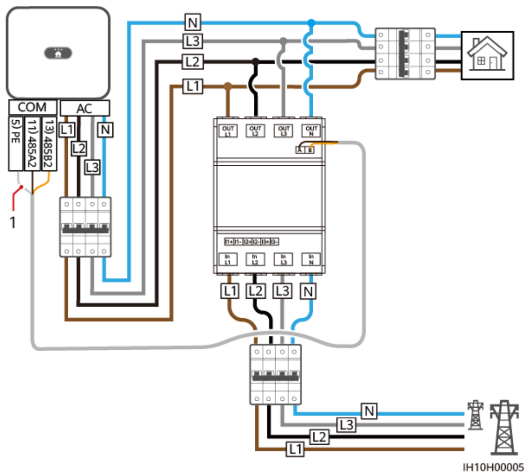
Afbeelding5-25 Driefasige, vierdraadse directe aansluiting (Smart Dongle-netwerk)
