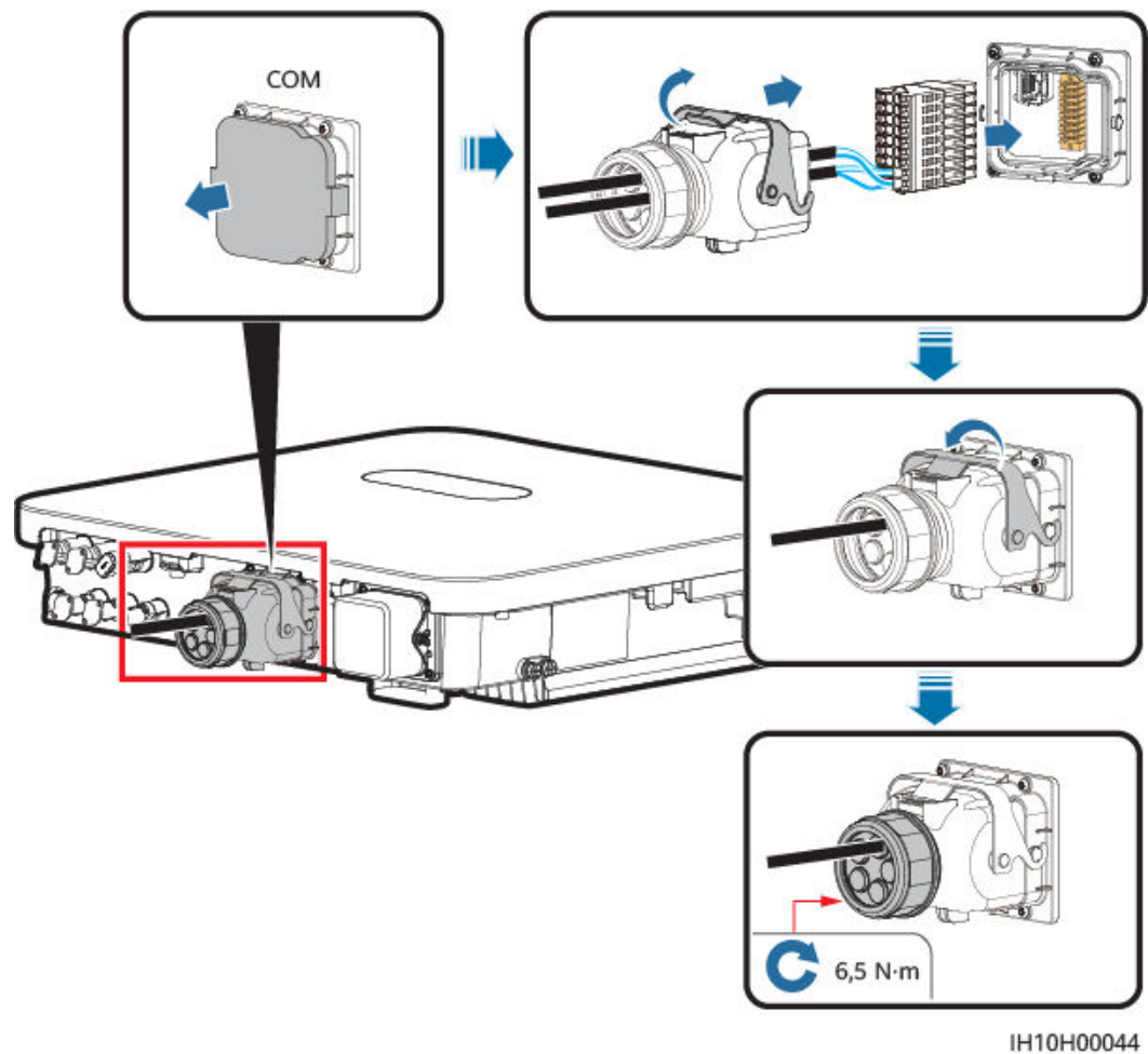
Afbeelding5-40 De aansluiting van de signaalkabel vastzetten
