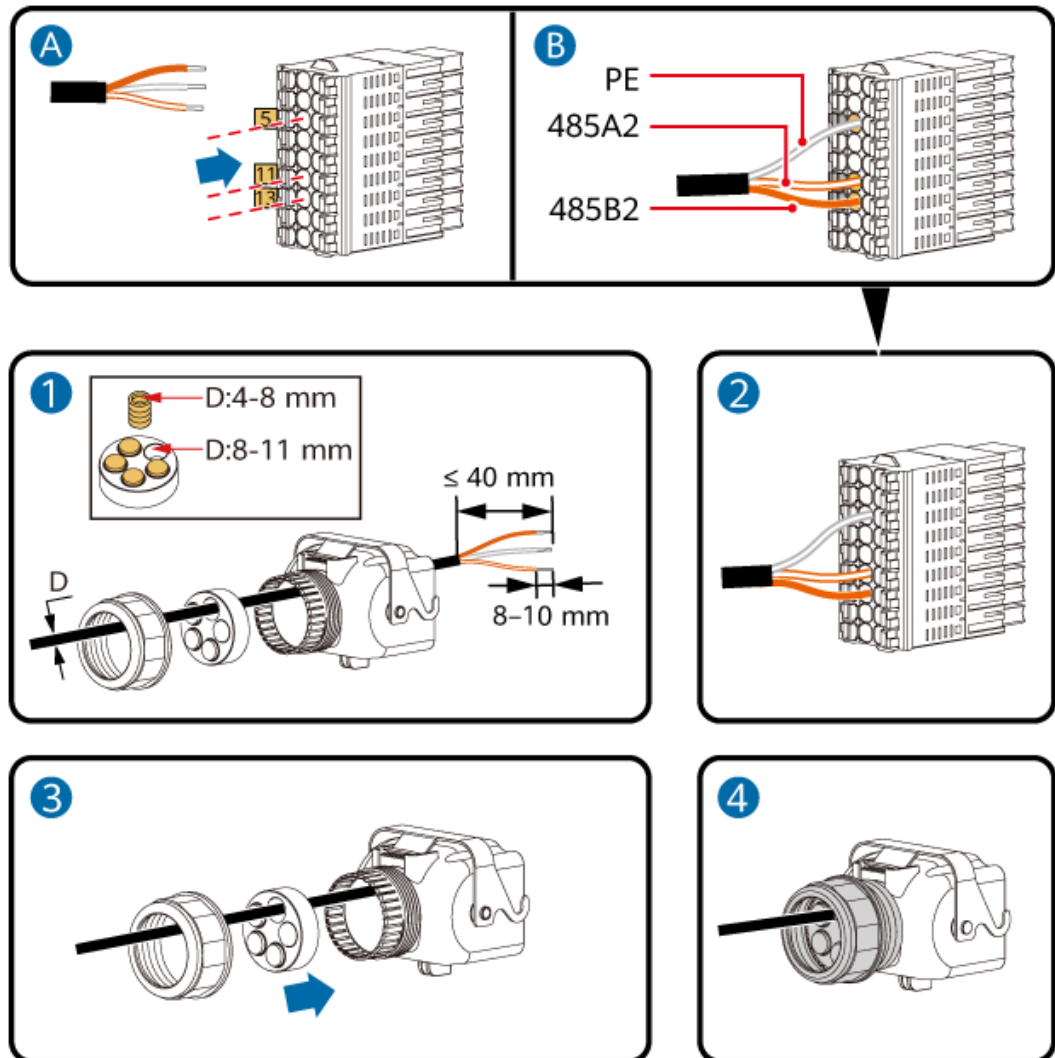
Afbeelding5-26 De kabel installeren
