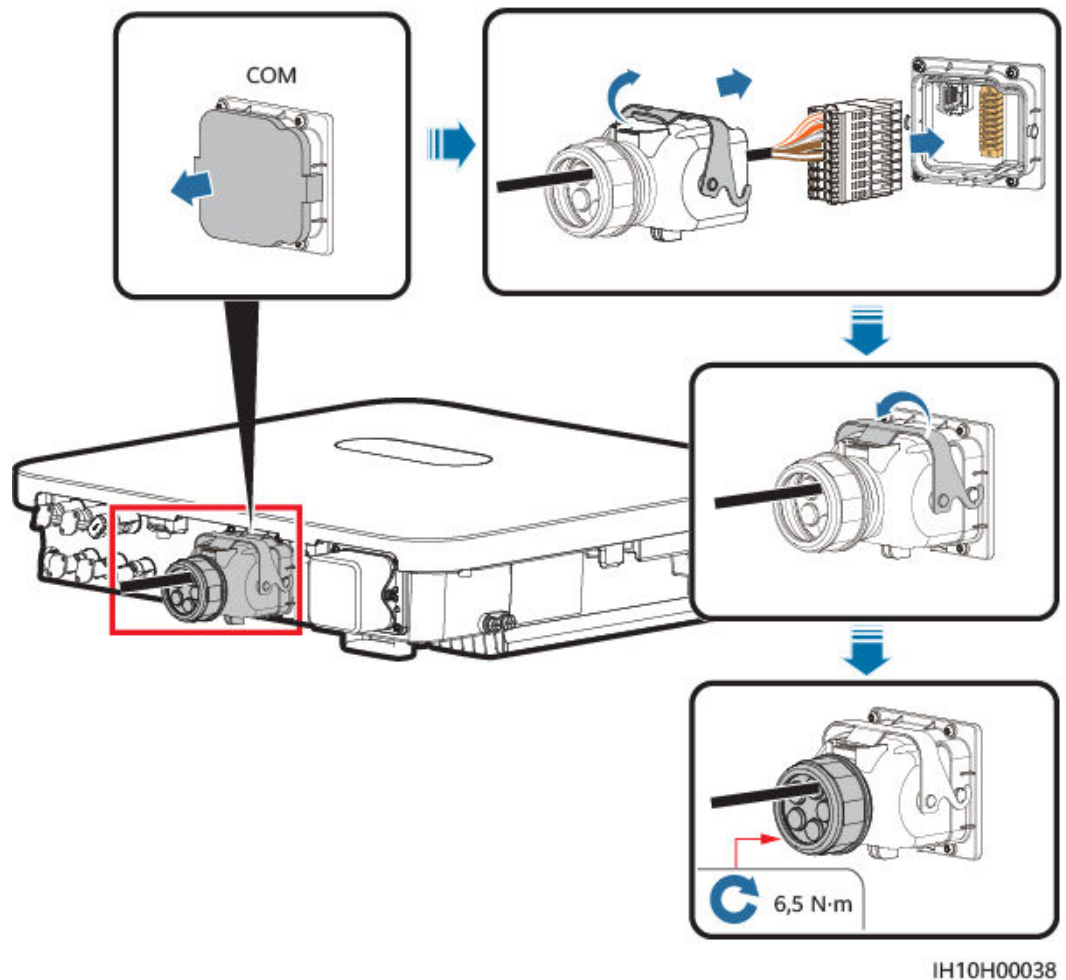
Afbeelding5-31 De aansluiting van de signaalkabel vastzetten
