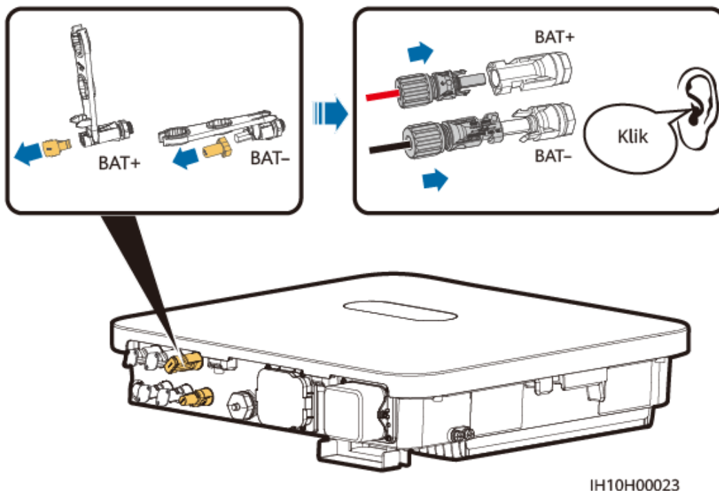
Afbeelding5-12 Batterijkabels aansluiten
