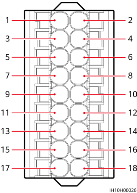
Afbeelding5-13 COM: 18-pins aansluiting
