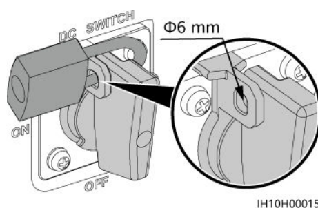
Afbeelding4-12 Een slot voor de DC-schakelaar installeren
