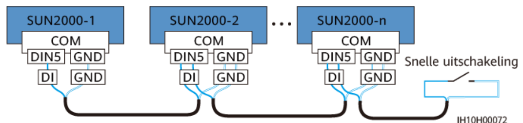
Afbeelding5-32 Gecascadeerde omvormers aansluiten op de schakelaar voor snelle uitschakeling
