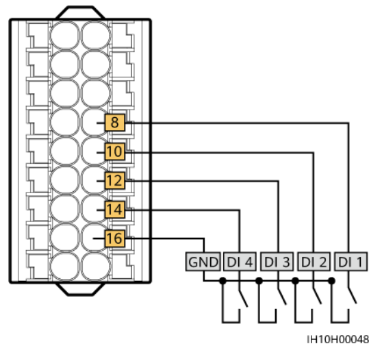
Afbeelding5-35 Kabelaansluiting
