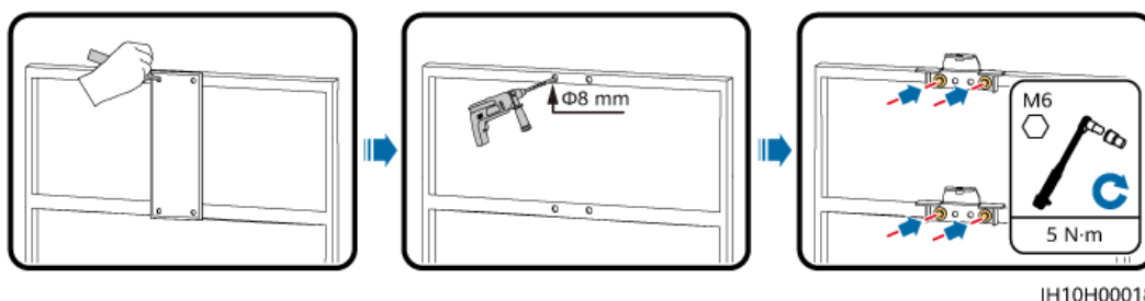
Afbeelding4-11 De montagesteunen installeren
