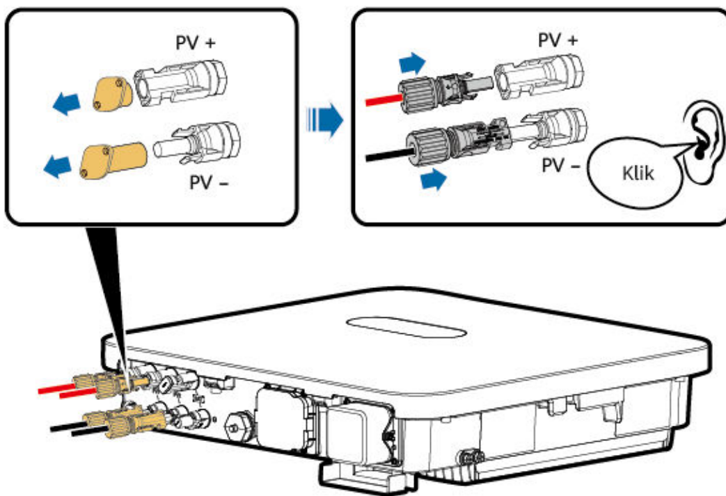
Afbeelding5-10 DC-ingangskabels aansluiten
