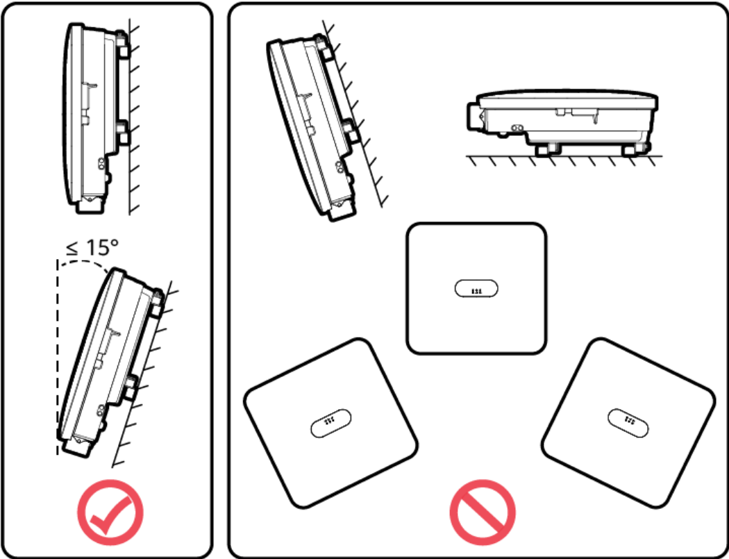
Afbeelding4-5 Installatiehoek
