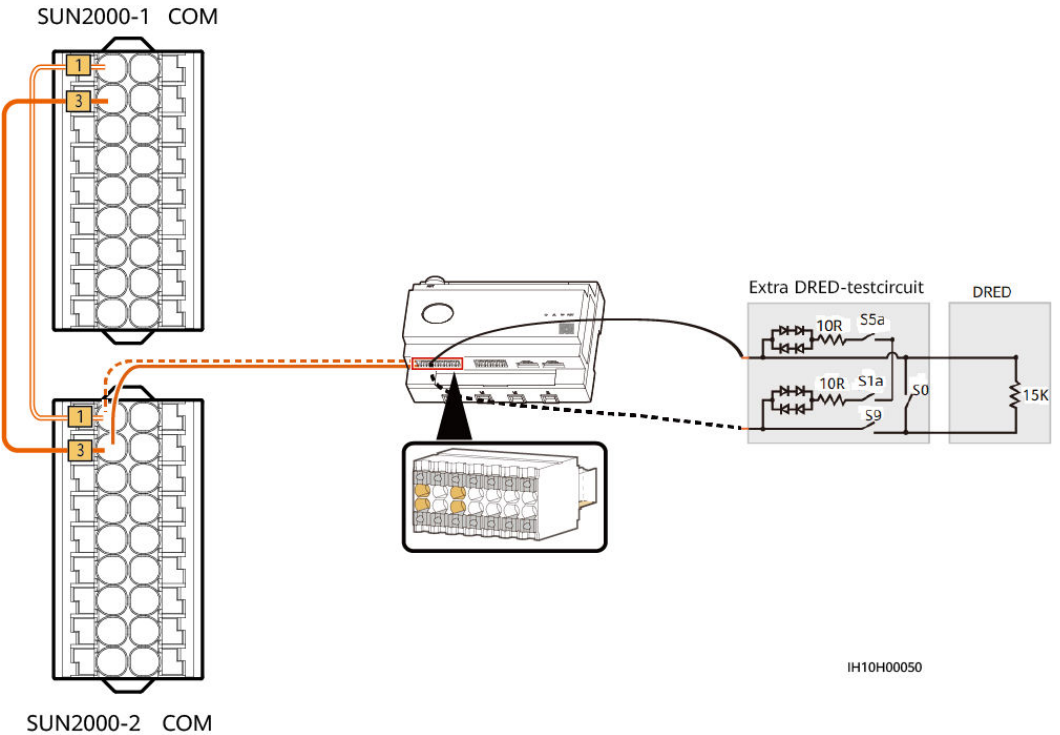
Afbeelding7-9 Aansluitschema voor de DRM-functie (EMMA-netwerk)
