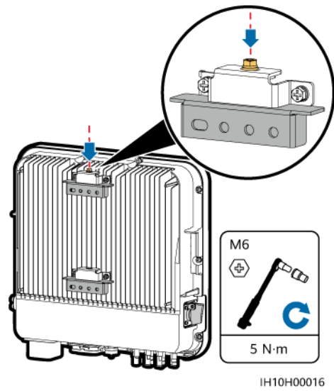
Afbeelding4-13 De omvormer installeren
