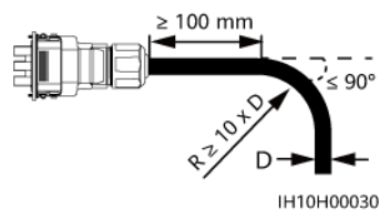
Afbeelding5-6 Bekabelingsvereisten
