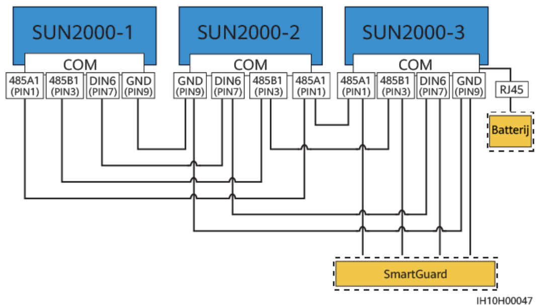
Afbeelding5-17 SmartGuard-netwerk (de onderdelen in kaders met een stippellijn rond zijn optioneel)
