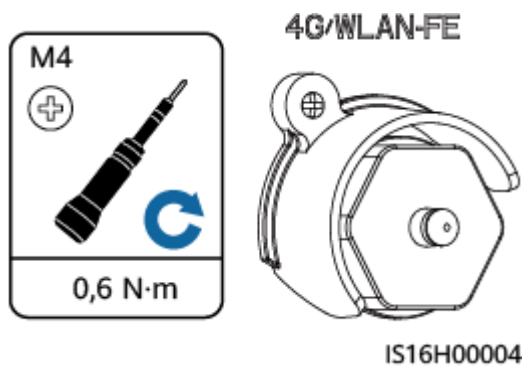
Afbeelding5-45 Antidiefstalonderdelen installeren voor de Smart Dongle
