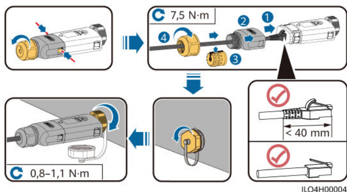
Afbeelding5-43 Een WLAN-FE Smart Dongle (FE-communicatie) installeren
