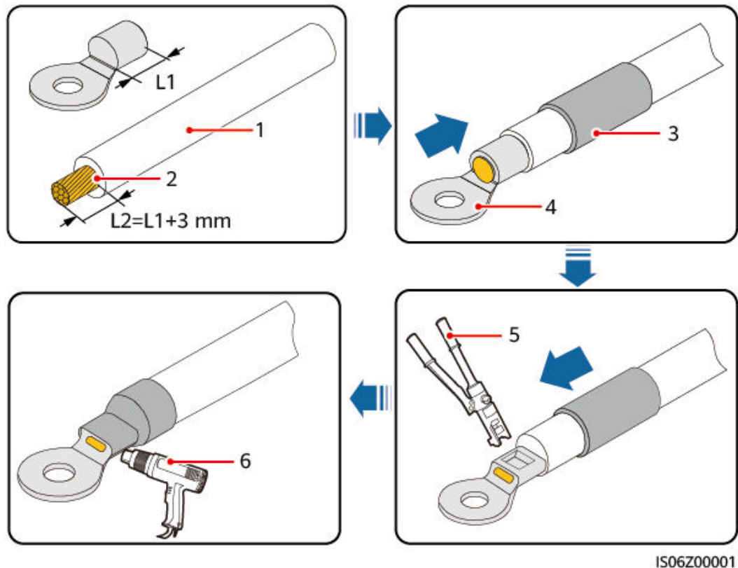
Afbeelding5-2 Een OT-aansluiting krimpen
