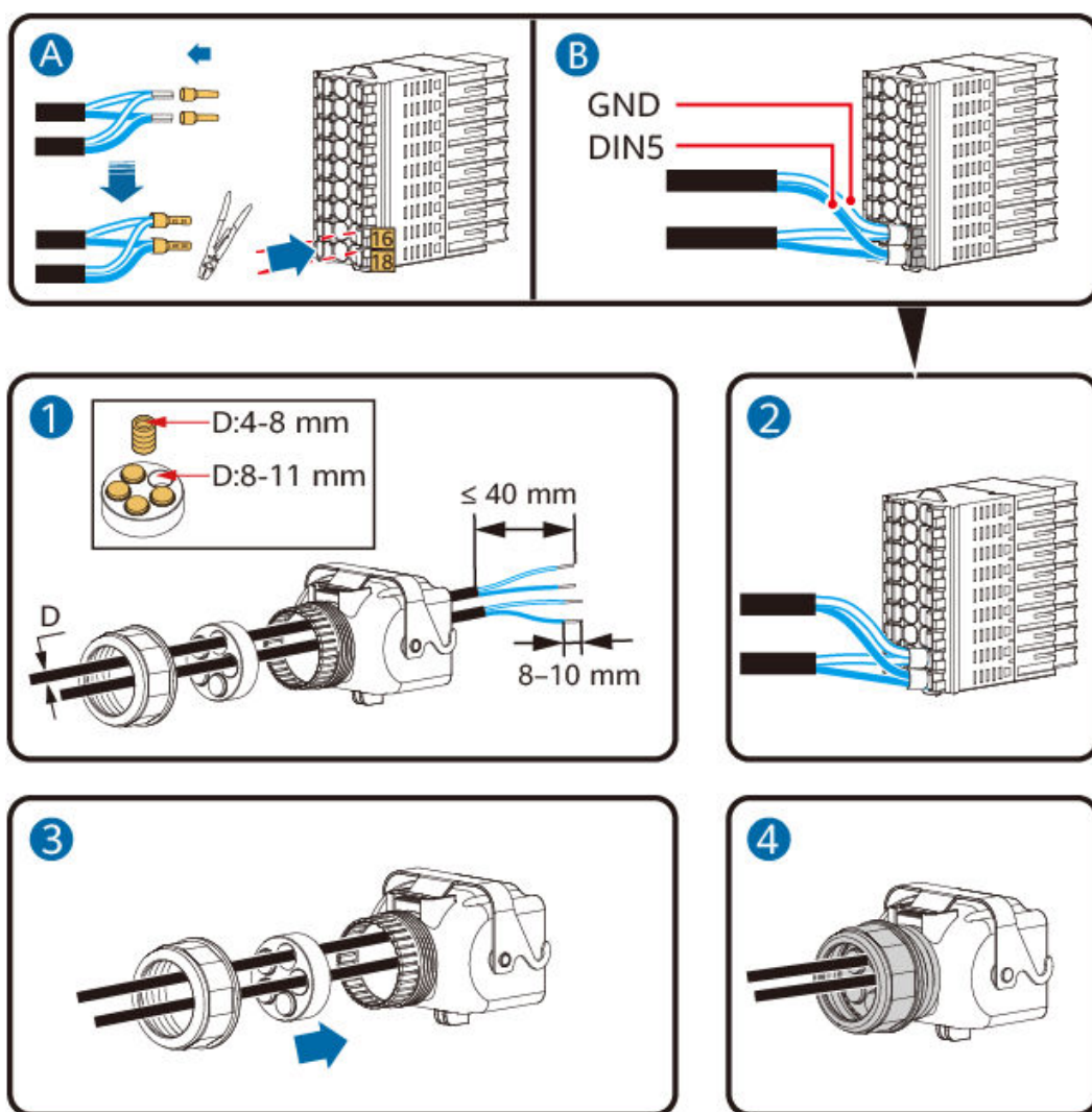
Afbeelding5-33 De kabel installeren
