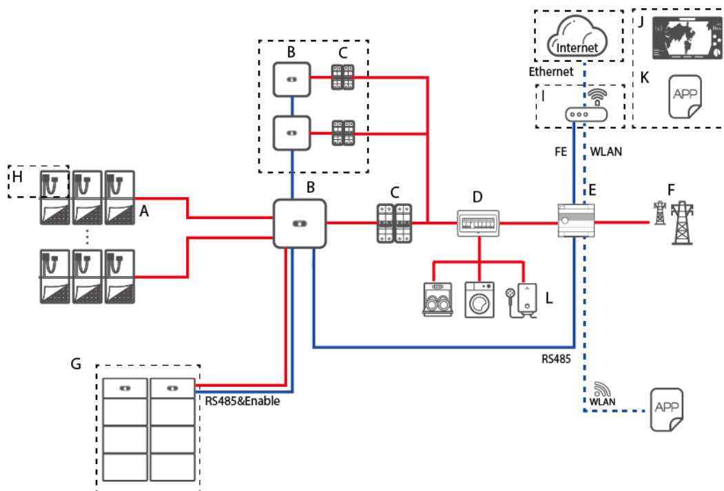
Afbeelding2-3 EMMA-netwerk (de onderdelen in kaders met een stippellijn zijn optioneel)
