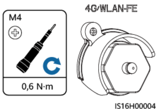
Afbeelding5-44 Antidiefstalonderdelen installeren voor de Smart Dongle
