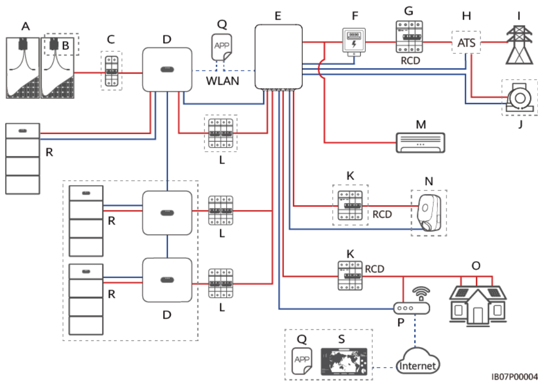
Afbeelding2-5 Netwerken waarvan enkele belastingen op de SmartGuard zijn aangesloten (kaders met een stippellijn geven optionele onderdelen aan)
