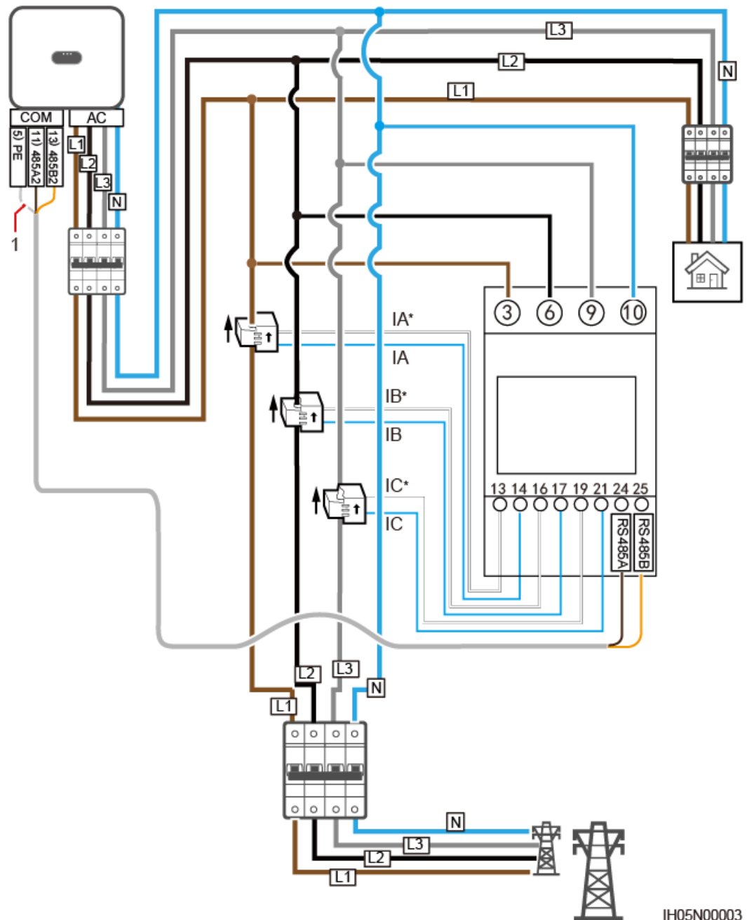
Afbeelding5-23 Driefasige, vierdraadse aansluiting (Smart Dongle-netwerk)
