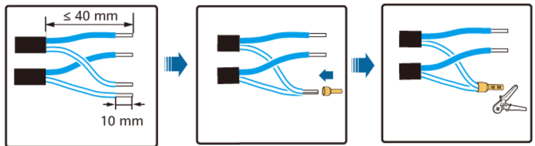
Afbeelding5-18 Twee signaalkabels krimpen
