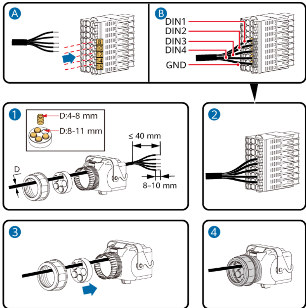
Afbeelding5-36 De kabel installeren
