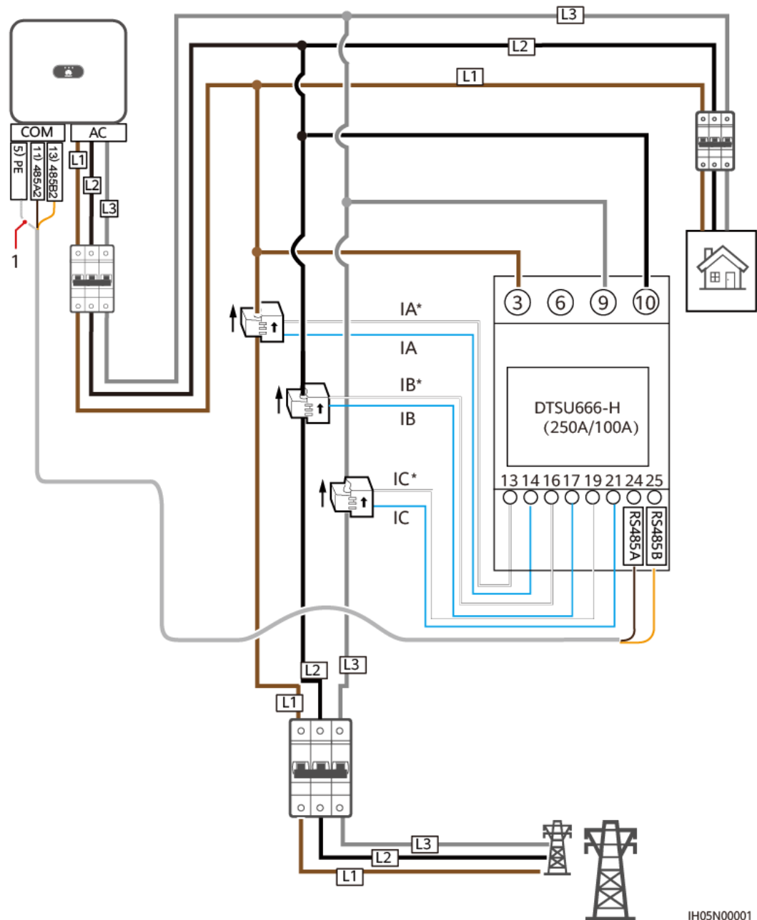
Afbeelding5-21 DTSU666-H (250 A/100 A) driedfasige, driedraadse kabelaansluiting (Smart Dongle-netwerk)
