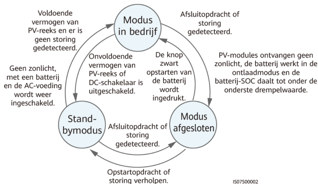
Afbeelding2-8 Werkmodi
