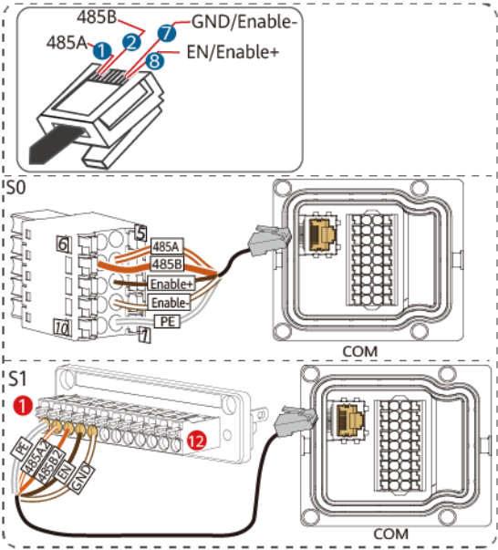
Afbeelding5-41 Kabelaansluiting
