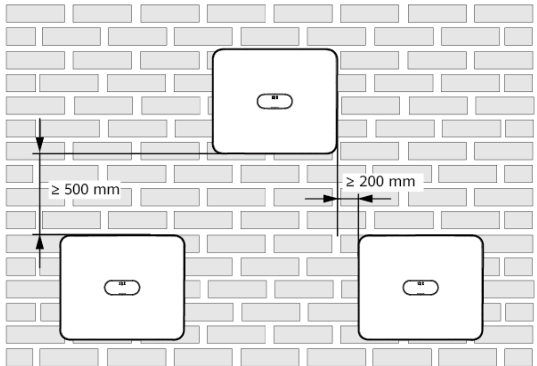
Afbeelding4-4 Driehoeksinstallatiemodus (aanbevolen)
