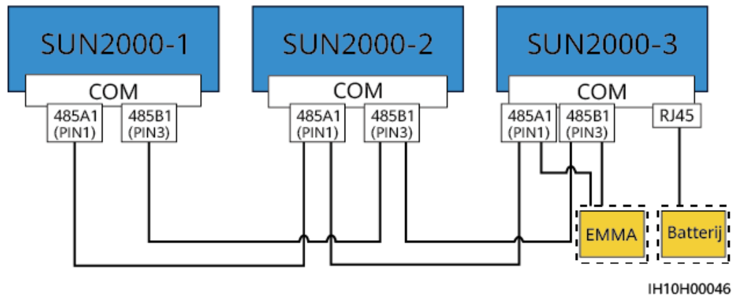
Afbeelding5-16 EMMA-netwerk (de onderdelen in kaders met een stippellijn zijn optioneel)
