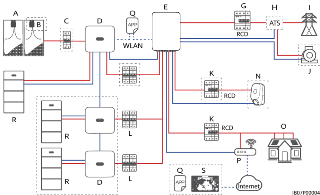
Afbeelding2-4 Netwerken waarvan alle belastingen op de SmartGuard zijn aangesloten (kaders met een stippellijn geven optionele onderdelen aan)
