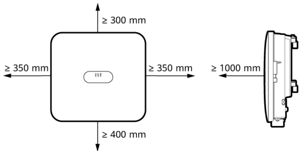
Afbeelding4-2 Vrije ruimte
